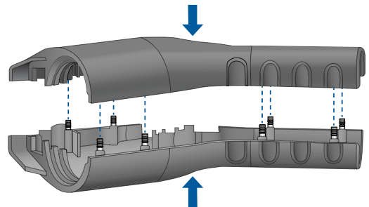
응용 예 : 전기 자동차 충전 핸들의 Press-N-Lok™ 핀
